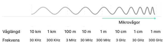
Figur 6: Illustration över en våglängds storlek vid olika frekvenser
